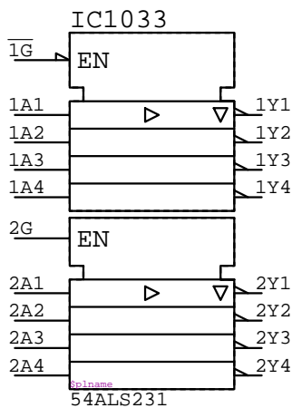
54ALS231
