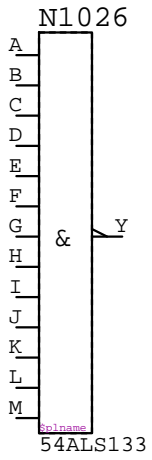
54ALS133 N????
