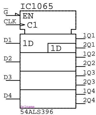
54ALS396
