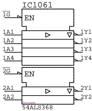
54ALS368
