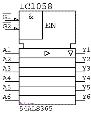
54ALS365
