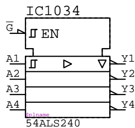
54ALS240
