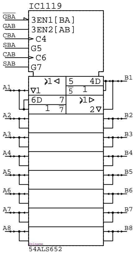
54ALS652
